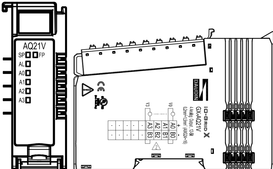
Figure 4.21 GX-AQ21V Wiring Diagram
